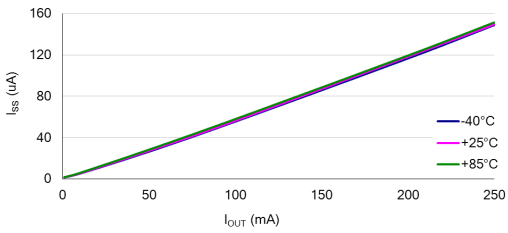
I_{SS} vs I_{OUT} : HT7333-2 ( V_{IN}=5.3V )
