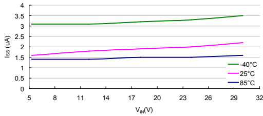
I_{SS} vs V_{IN} : HT75E33 ( I_{OUT}=0mA )
