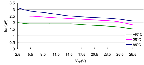
I_{SS} vs V_{CE} : HT75E50 ( I_{OUT}=0mA )
