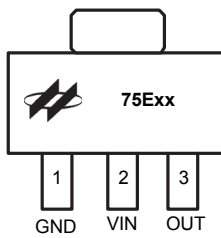
SOT89-3
