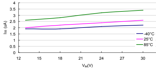
I_{SS} vs V_{IN} : HT75EC0 ( I_{OUT}=0mA )
