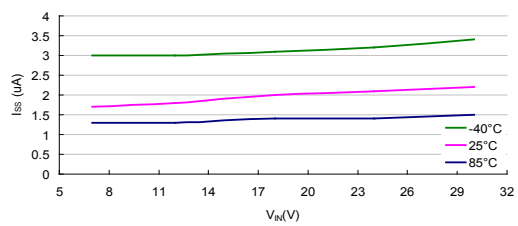
I_{SS} vs V_{IN} : HT75E50 ( I_{OUT}=0mA )
