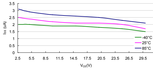
I_{SS} vs V_{CE} : HT75E60 ( I_{OUT}=0mA )
