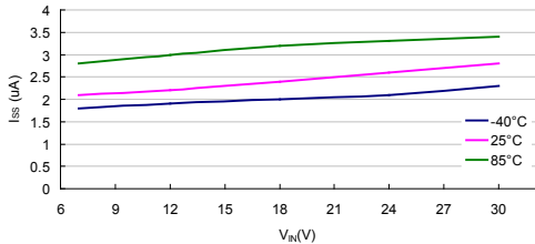
I_{SS} vs V_{IN} : HT75E60 ( I_{OUT}=0mA )
