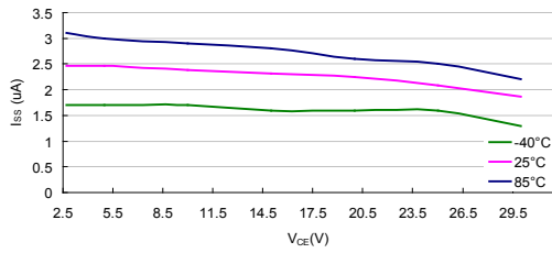
I_{SS} vs V_{CE} : HT75E33 ( I_{OUT}=0mA )
