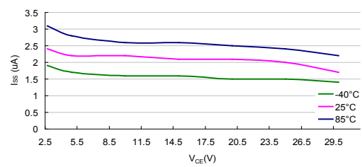
I_{SS} vs V_{CE} : HT75EC0 ( I_{OUT}=0mA )
